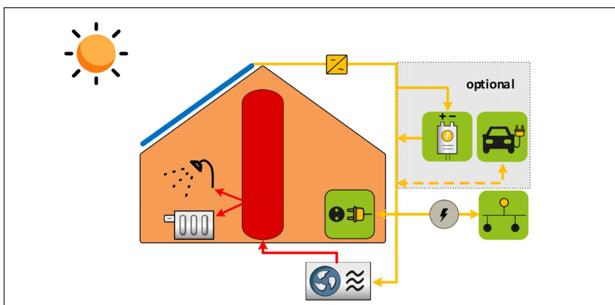
Bild 5: Sonnenhaus mit Photovoltaik und Wärmepumpe
