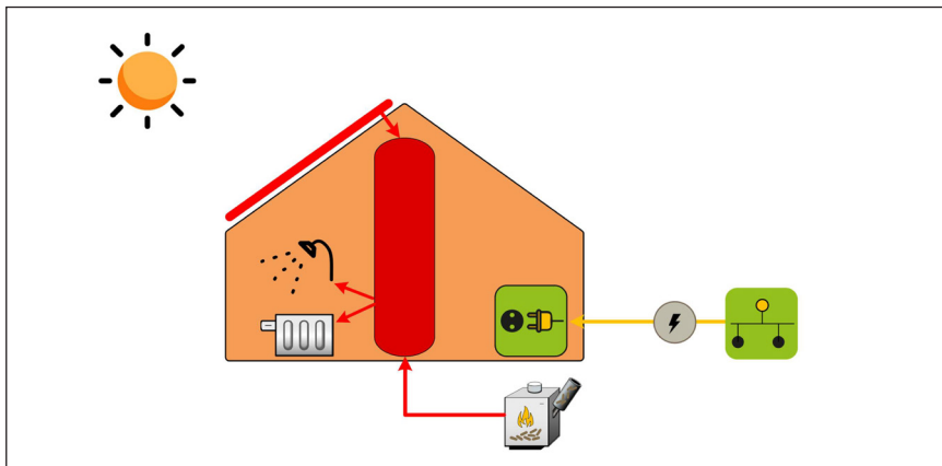
Bild 4: Klassisches Sonnenhaus mit Biomasseheizung
