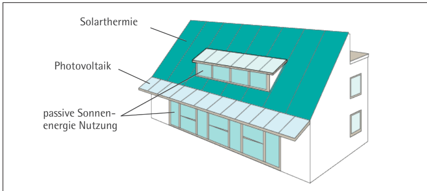
Bild 1: Energetisch effektive Solararchitektur bedeutet, dass überschüssiger Solarstrom für die Elektromobilität und die Einspeisung ins öffentliche Netz genutzt werden kann. Daher sind etwas flachere Neigungswinkel für PV-Module, im Vergleich zu den Solarthermie-Kollektoren, sinnvoll, und größere Südabweichungen wirken sich weniger negativ aus
