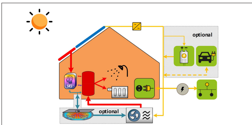
Bild 7: Sonnenhaus Hybrid mit Sonnenhaus-Kompakt-System
